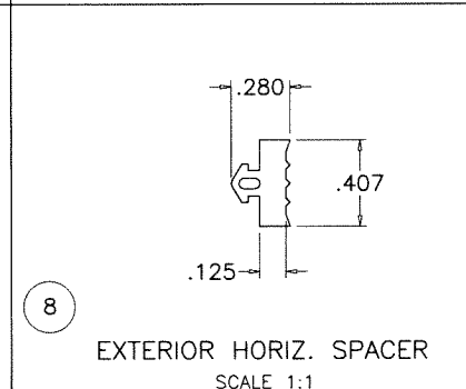
7 EXTERIOR VERT. SPACER SCALE 1:1
